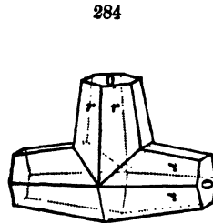
Pyrrhotite.
